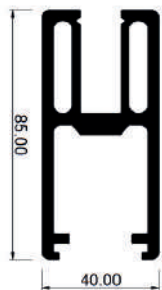
Zócalo
