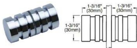
Pomo
