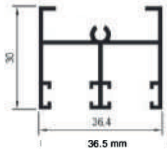
Cabezal 2 Canales
