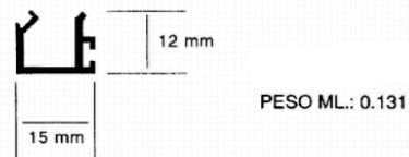
Pisa Vidrio
