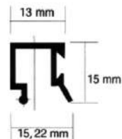
Pisavidrio
