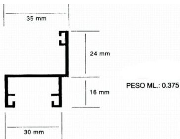
Perfil Marco
