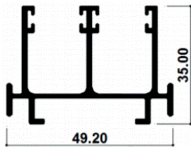
Cabezal 2 Canales
