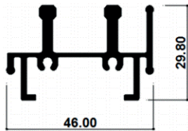
Cabezal 2 Canales
