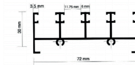
Cabezal 4 Canales
