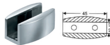
Guía - Piso
