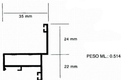
Perfil Hoja
