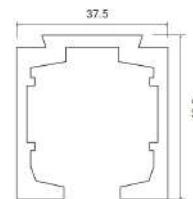
Cabezal - Riel
