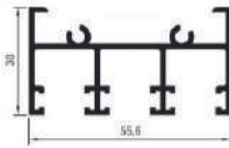
Cabezal 3 Canales
